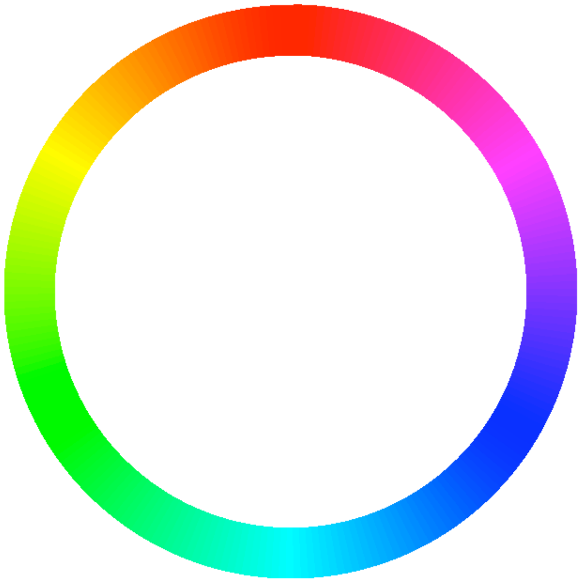
Cercle chromatique
